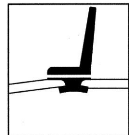
anextrudierte Dichtung GEALAN 610102
